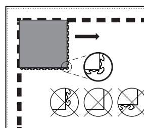
Fig. 3 Sens de pose des dalles INVISIBLE, INVISIBLE XL, BUSINESS
